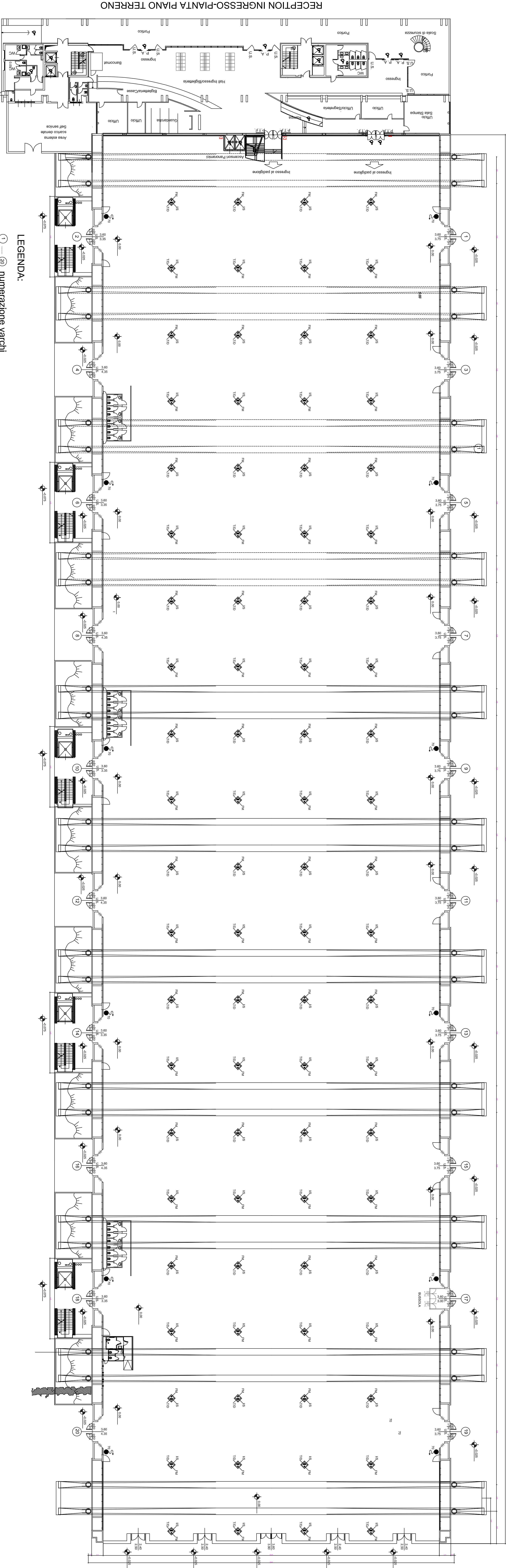
PADIGLIONE SUD-PIANTA PIANO TERRENO-Q. 0.00
